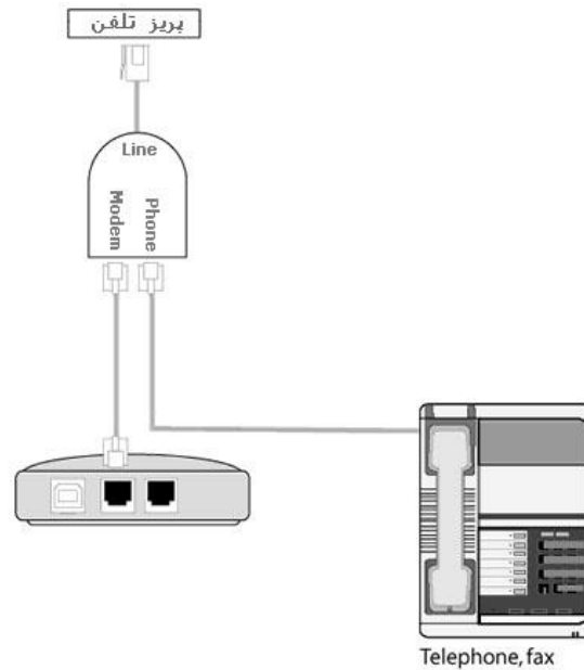
شکل ۲ - نحوه اتصالات اسپلیتر
